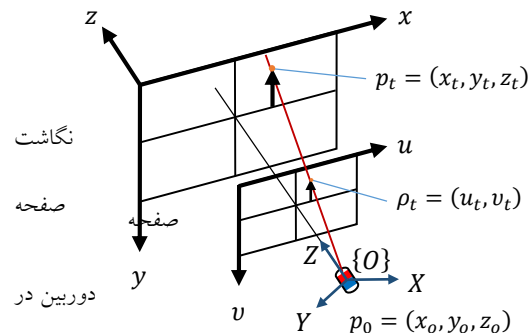
شکل (۳): مدل دوربین سوراخ‌سوزنی
